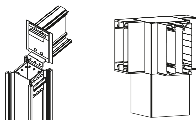
Σύνδεση κολόνας με ενδιάμεση τραβέρσα
