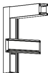
Σύνδεση προφίλ κολόνας και τραβέρσας
