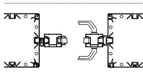
Λεπτομέρειες
