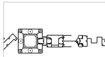
Λεπτομέρειες
